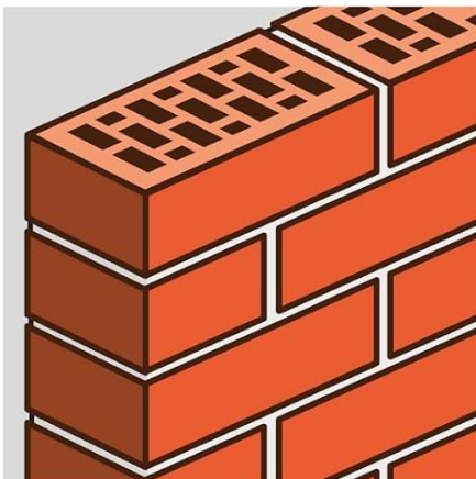
Muratura
